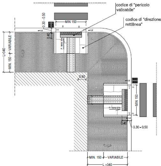
Pavimentazione in cubetti
