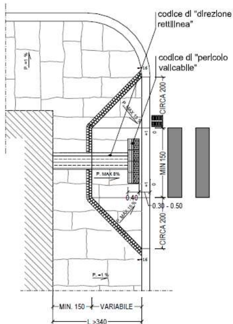
Pavimentazione in asfalto o lastre lapidee
