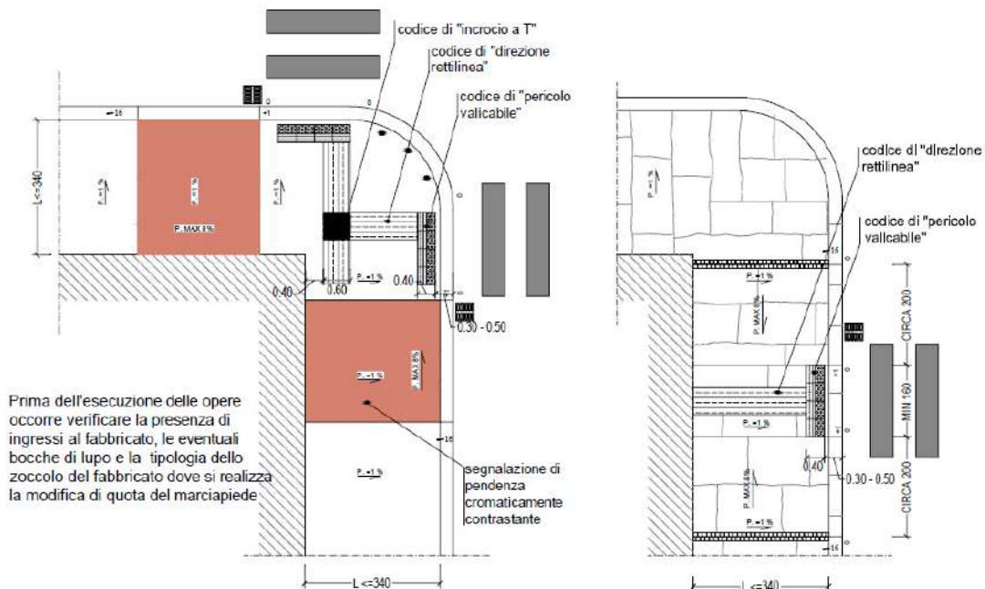
Pavimentazione in asfalto o lastre di pietre
